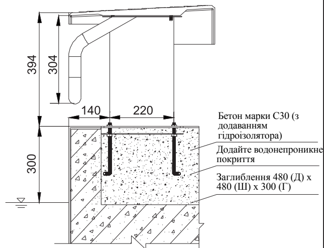
Схема установки (Одиниця виміру: мм)
